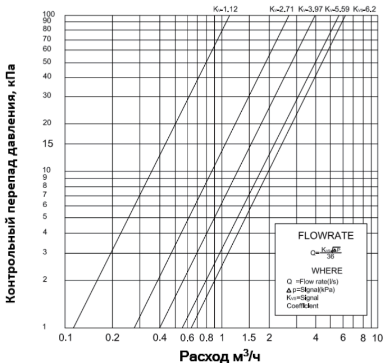
Клапан 1206 DN20
